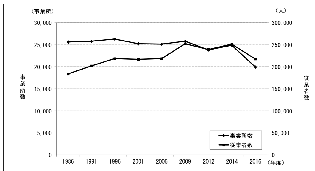
図3 鹿児島市における民生業務部門の事業所数と従業者数の推移
