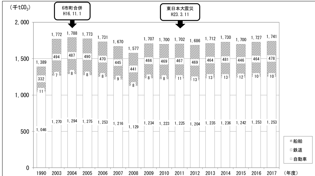
図6 運輸部門におけるCO 2 排出量の推移
