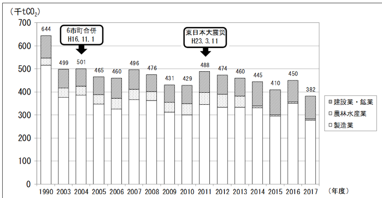
図 1 1 産業部門におけるCO 2 排出量の推移
