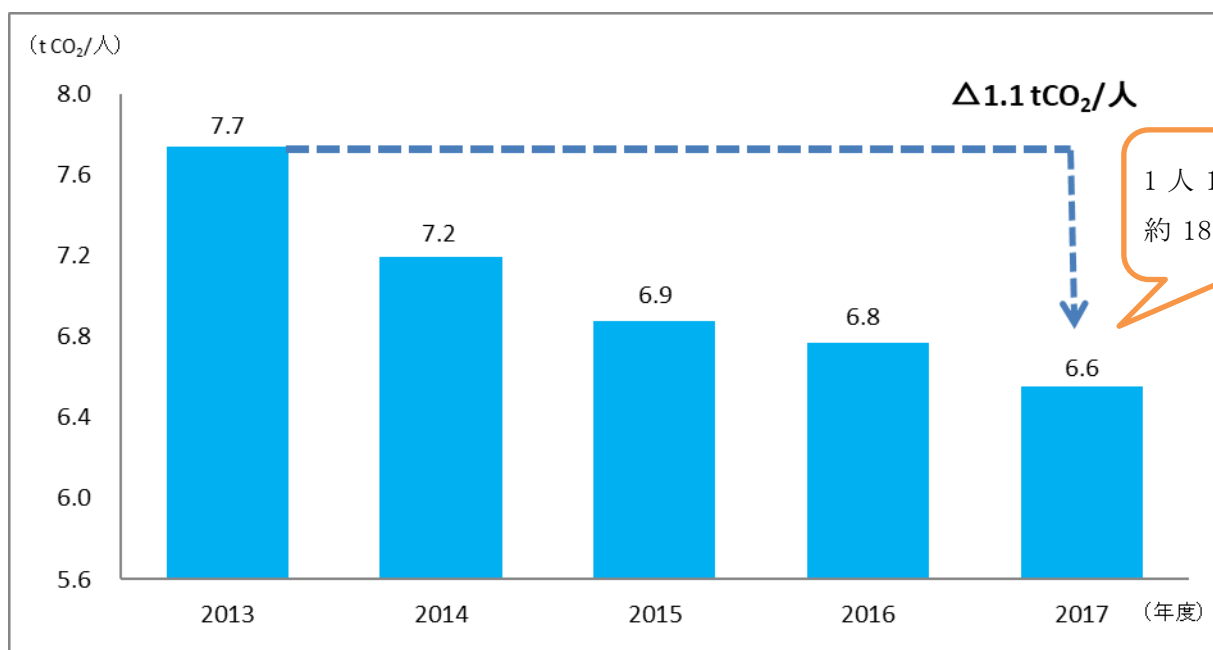
図2 市民1人当たりのCO 2 排出量
