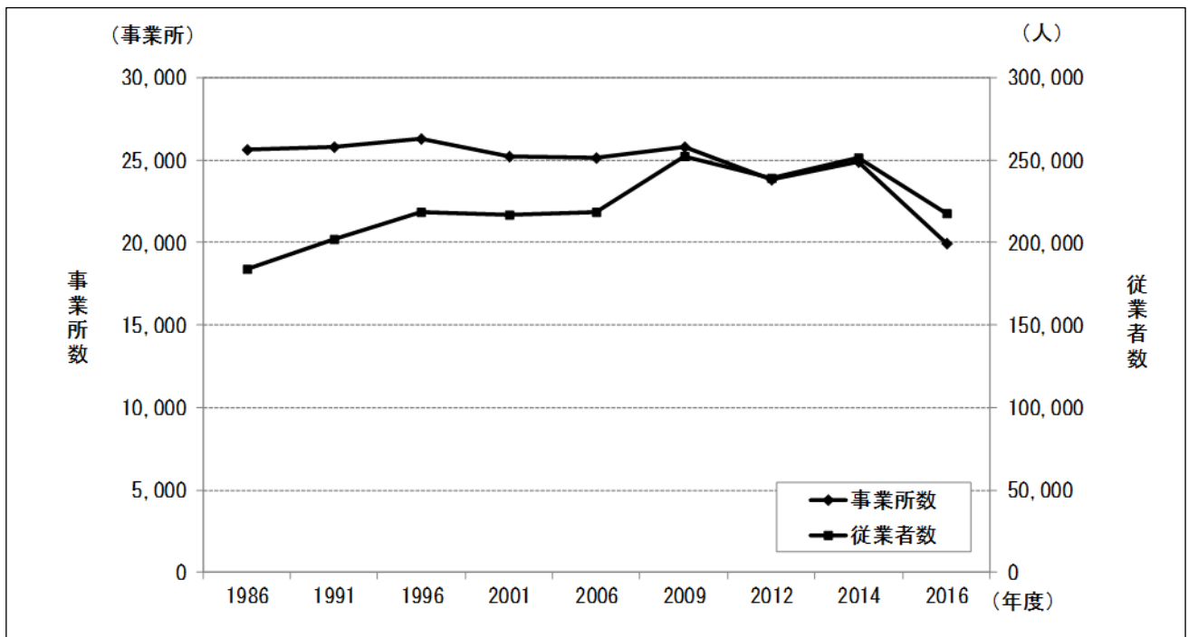
図10 鹿児島市における民生業務部門の事業所数と従業者数の推移
