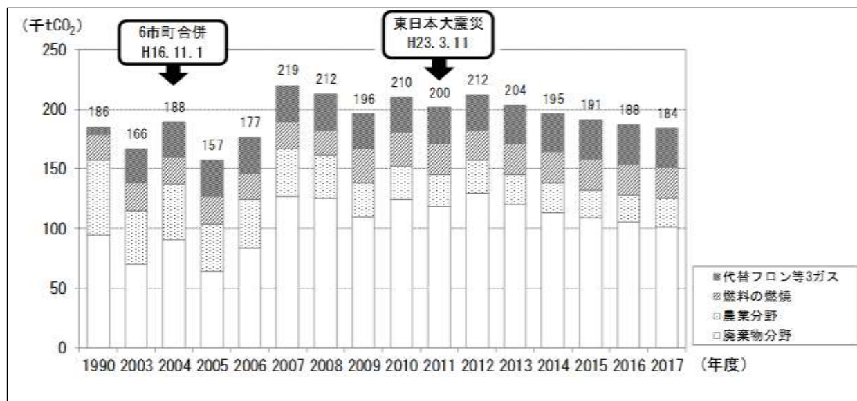
図13 その他部門におけるCO 2 排出量の推移
