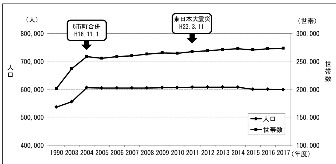
図８ 鹿児島市における人口と世帯数の推移
