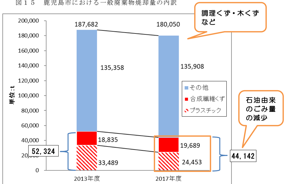
図 1 5 鹿児島市における一般廃棄物焼却量の内訳
