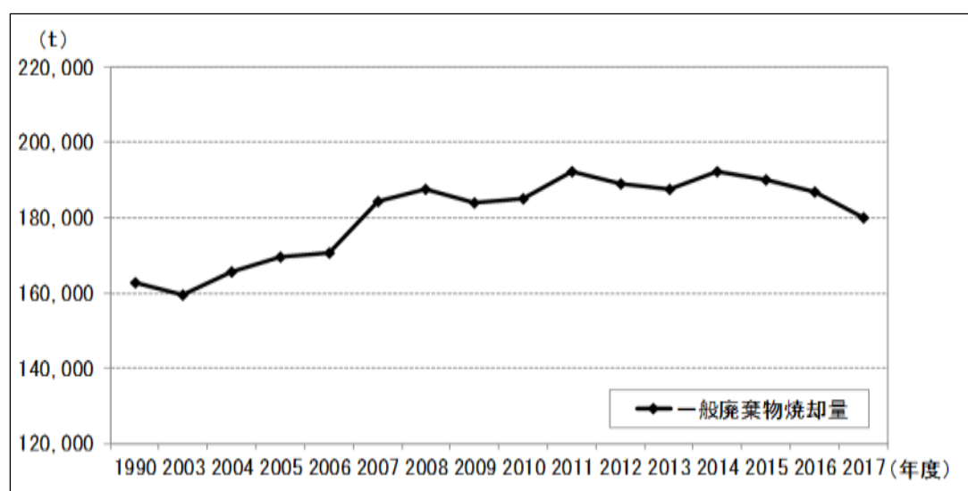
図14 鹿児島市における一般廃棄物焼却量の推移
