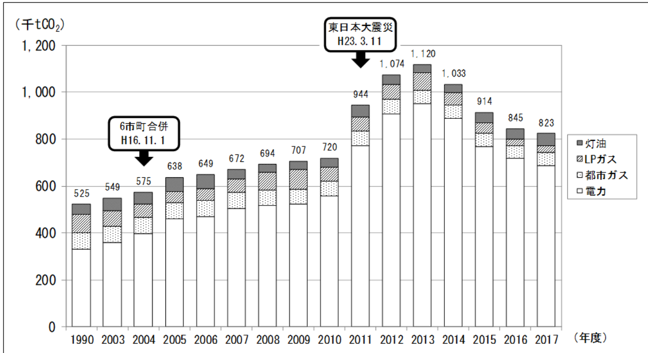
図７ 民生家庭部門におけるCO 2 排出量の推移
