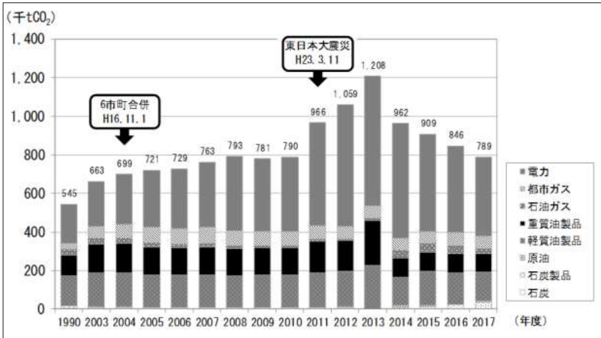
図9 民生業務部門におけるCO 2 排出量の推移
