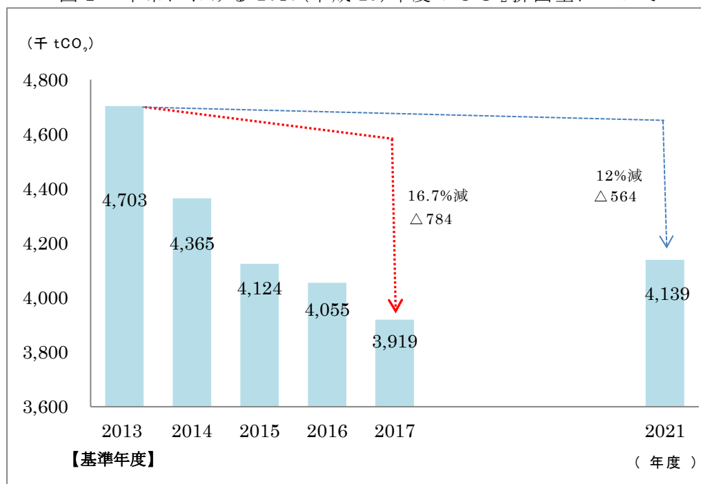
図1 本市における2017(平成29)年度のCO 2 排出量について
