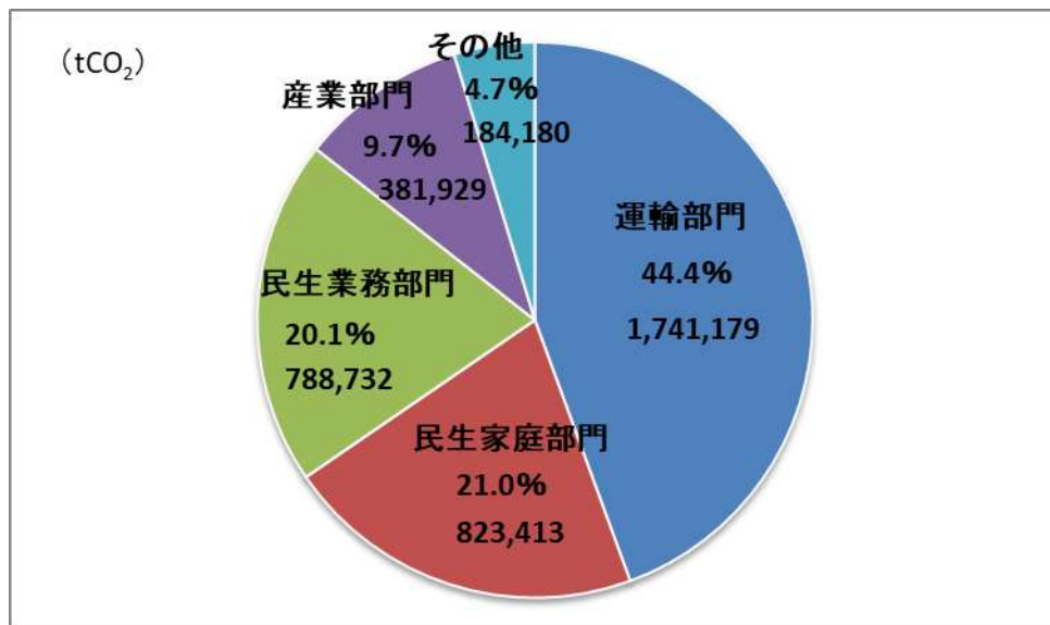
図5 CO 2 排出量の部門別内訳
