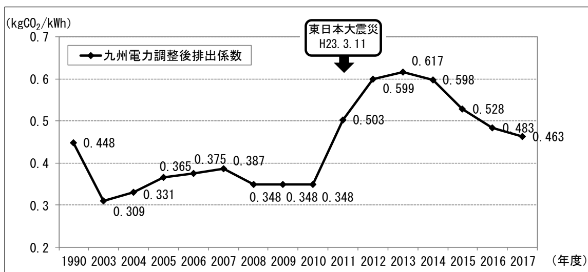
図4 排出係数の推移（九州電力管内）
