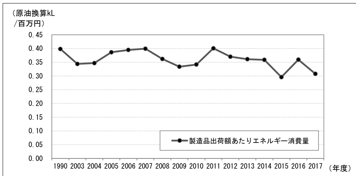
図 1 2 製造業における事業所数・製造品出荷額等の推移
