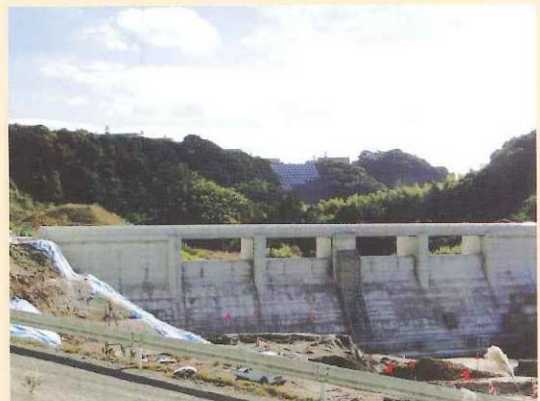
西之谷ダム(建設中) (平成25年4月供用開始予定)
