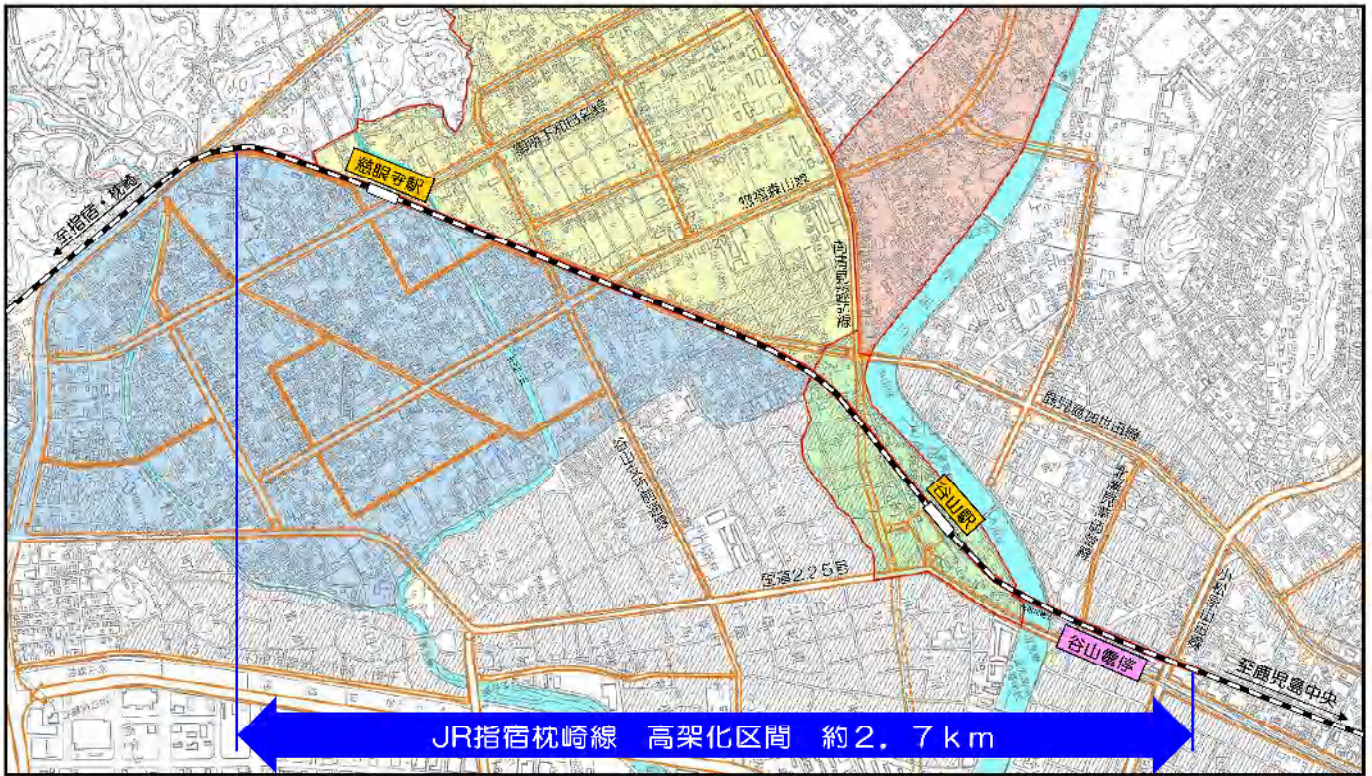
谷山地区連続立体交差事業全体図
