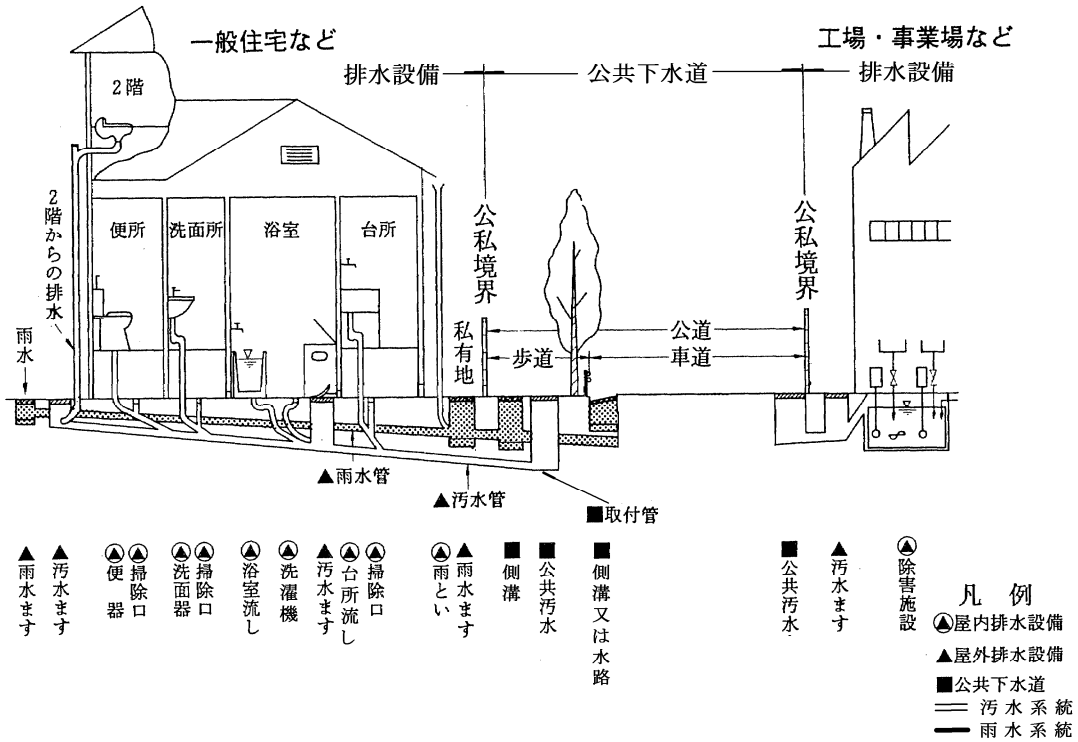
図 1-1 排水設備の例 (分流式)
