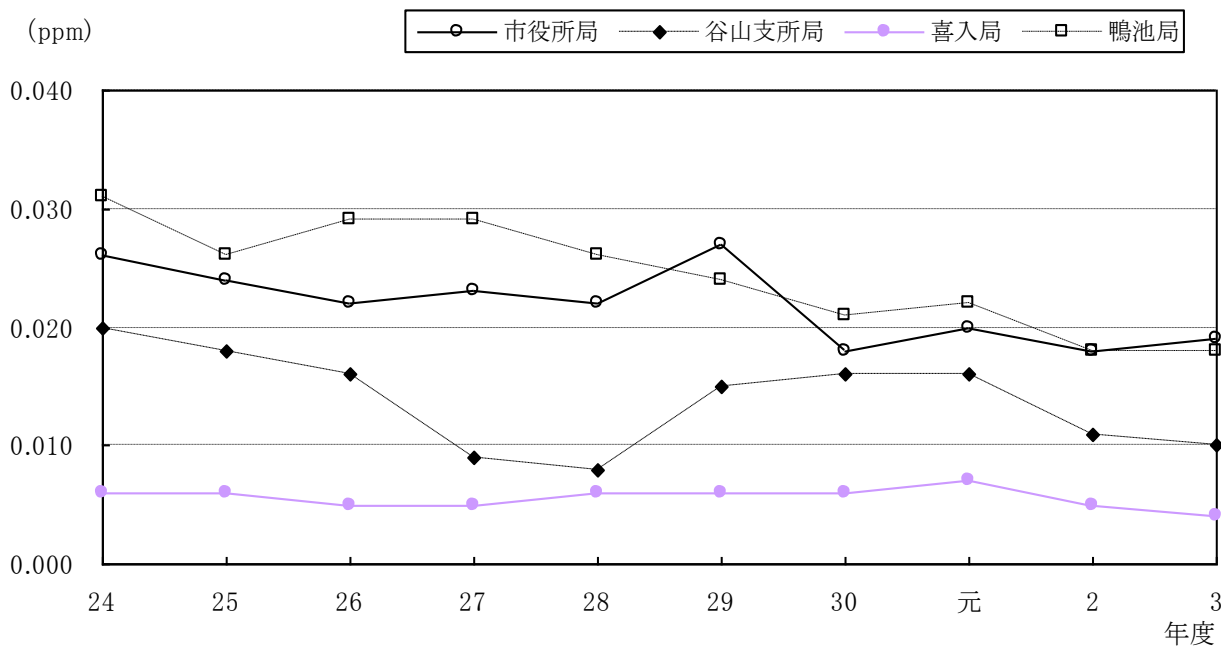
図 3-8 環境基準の長期的評価 (1日平均値の年間98%値) の経年変化
