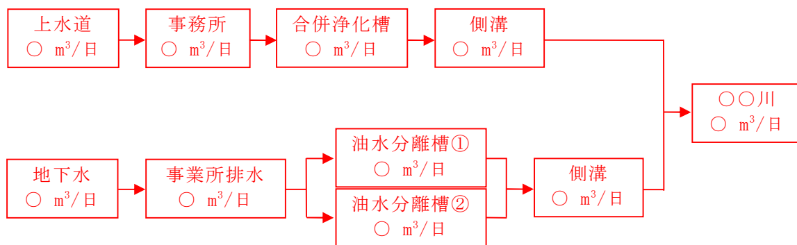
用水及び排水の系統説明図
