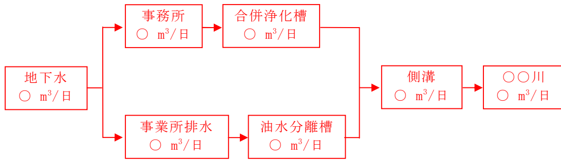
用水及び排水の系統説明図
