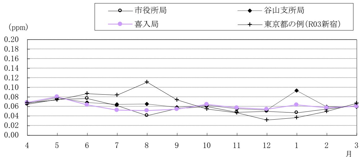
図 13 日最高値（昼間の 1 時間値）の月毎推移
