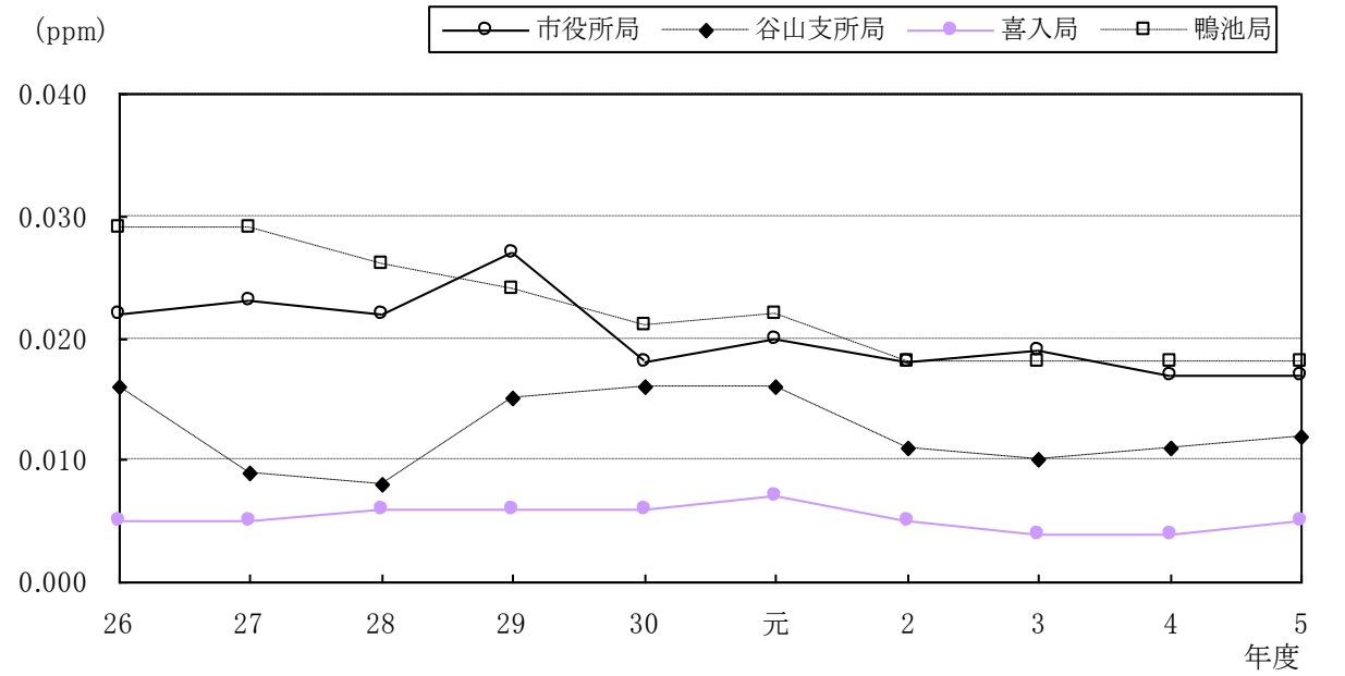
二酸化窒素の経年変化グラフ
