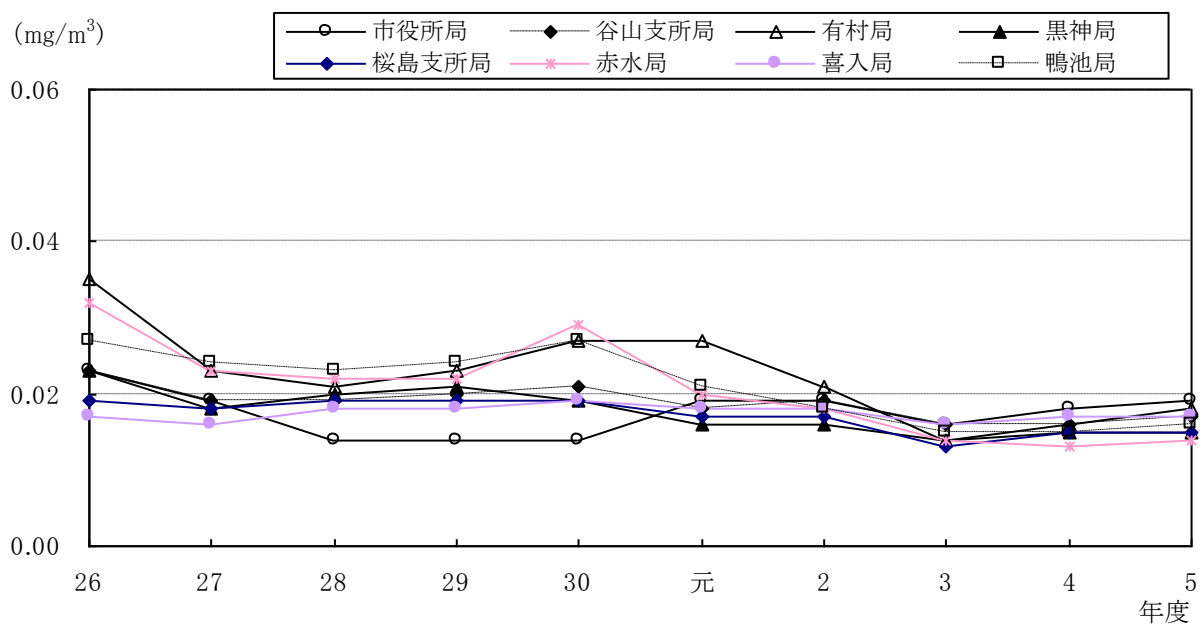
図4 1時間値の年平均値の経年変化
