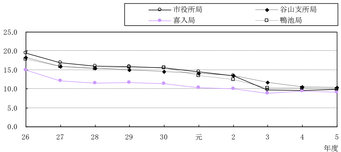
図5 環境基準の長期的評価(1年平均値)の経年変化
