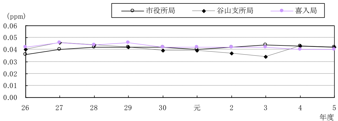
図 11 年平均値（昼間の日最高1時間値）の経年変化
