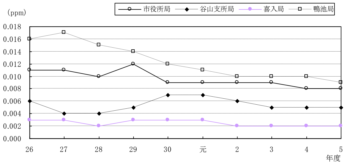
図9 1時間値の年平均値の経年変化
