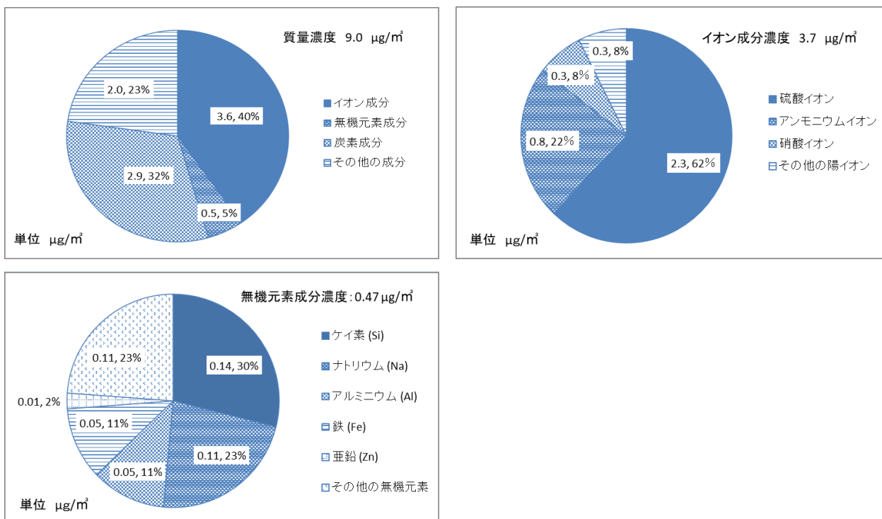
図7 微小粒子状物質の成分濃度 (令和5年度 年平均値)
