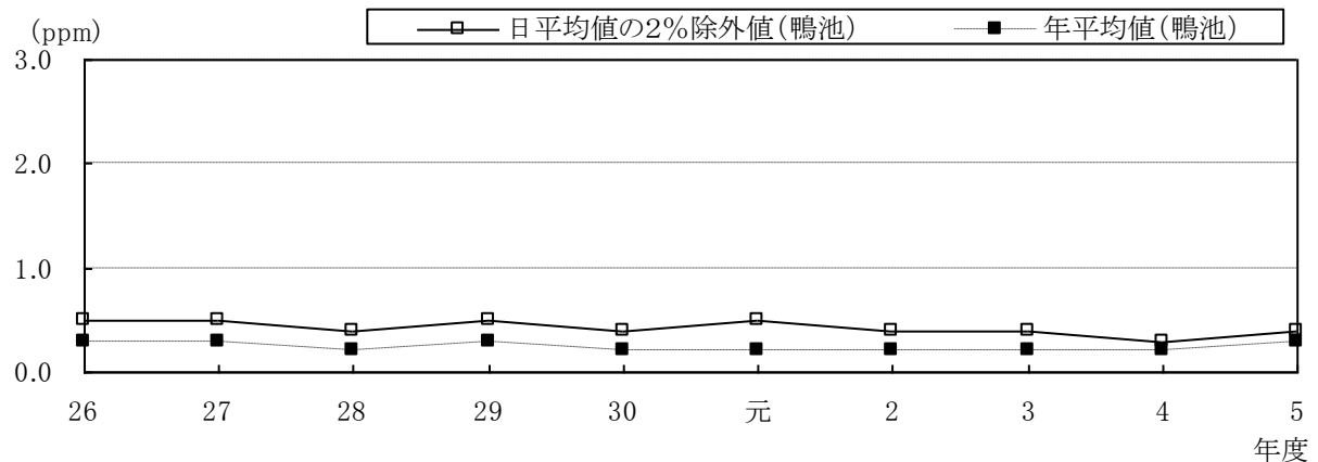
図 10 環境基準の長期的評価（1 日平均値の年間 2 % 除外値） 及び 1 時間値の年平均値の経年変化
