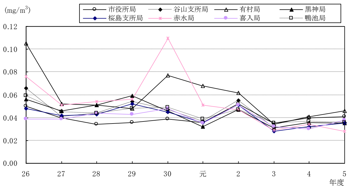
浮遊粒子状物質の経年変化グラフ
