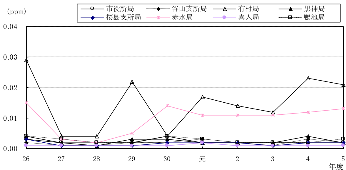
図 1 環境基準の長期的評価（1 日平均値の 2 % 除外値）の経年変化
