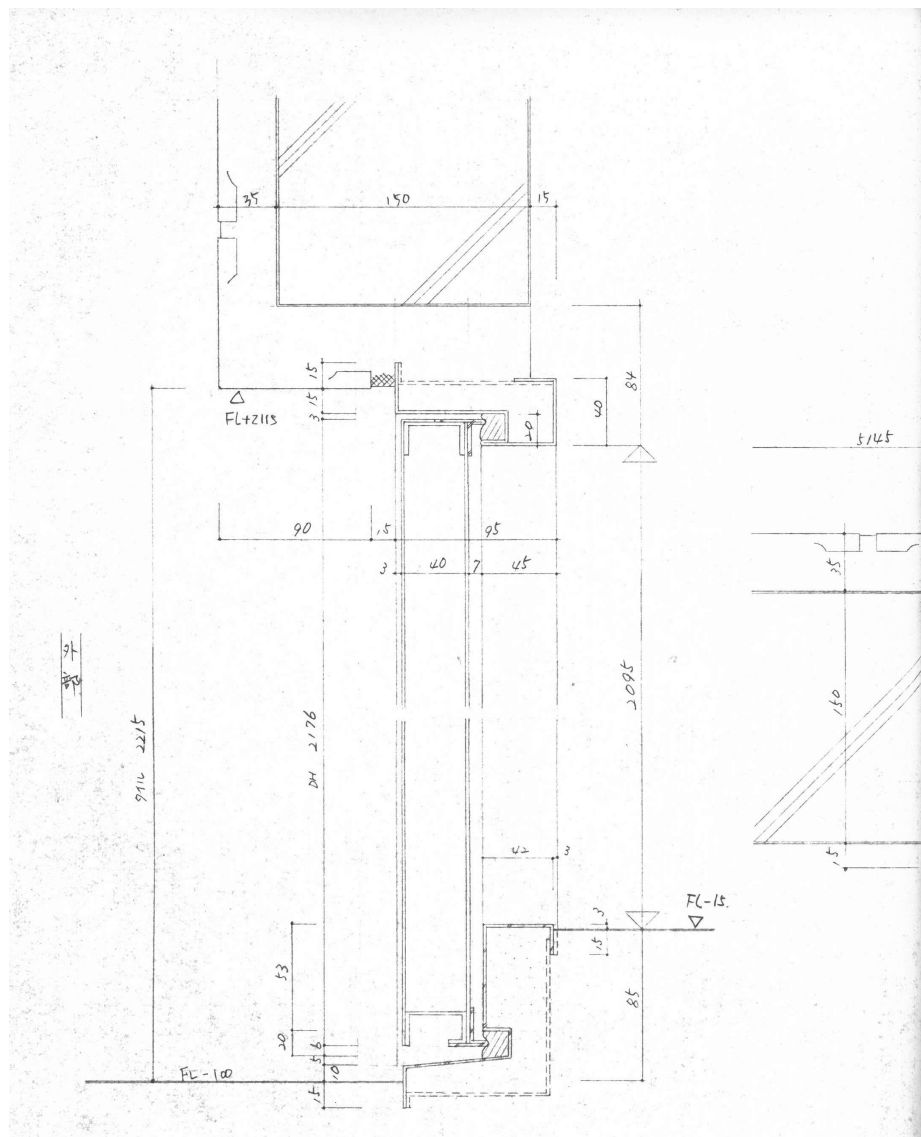
イルカ館調餌室現況図2 N.S.
