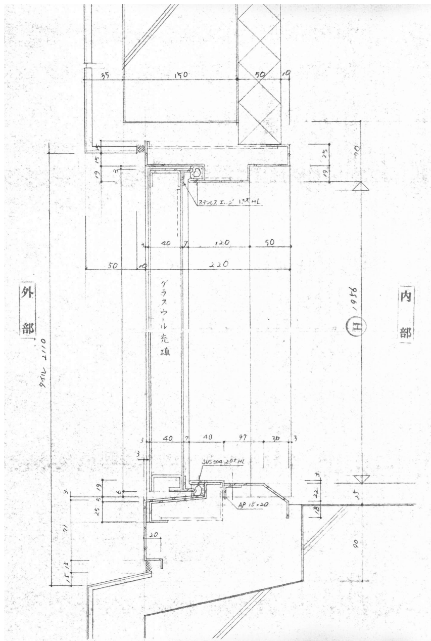
受水槽室断面図2 N.S.
