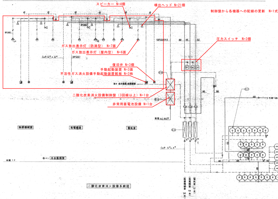
系統図 N.S.
