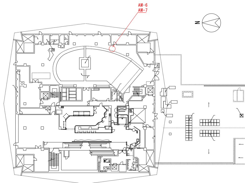
本館3階平面図 1/300
