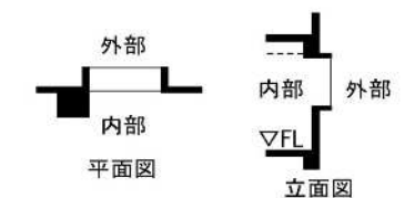
図 2. 床面積に算入されない場合
