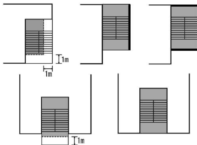
図3 2面以上壁に囲まれる場合
