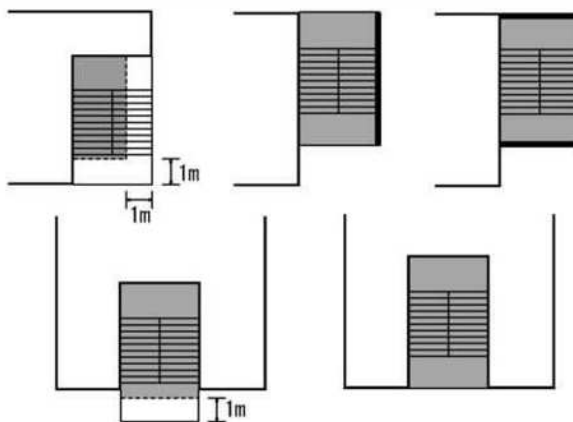
図3 2面以上壁に囲まれる場合
