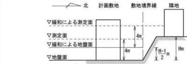
図1 高低差による緩和・日影の測定面の位置
