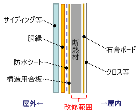
図2-1 横から見た断面図
