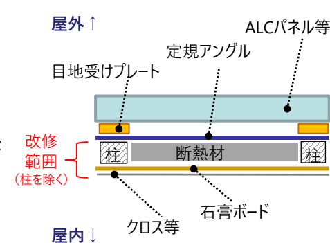
図2-4 上から見た断面図
