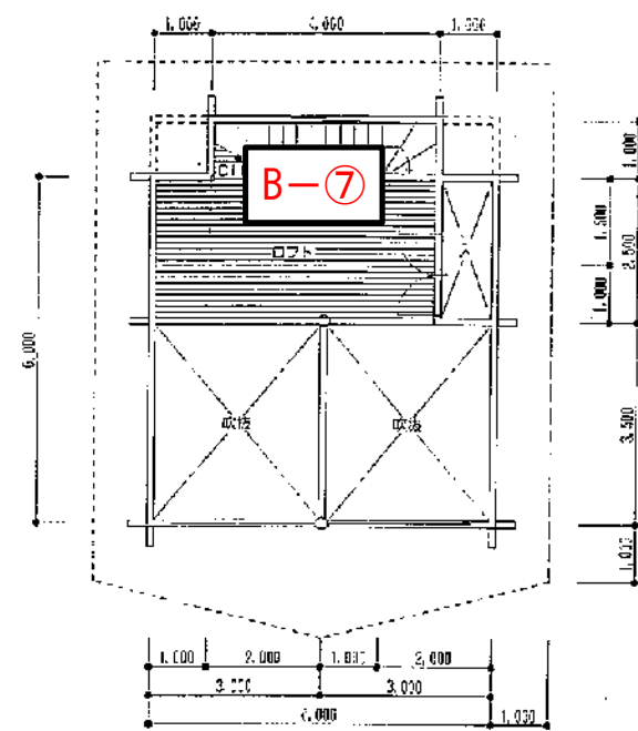
2階平面図 S=1:100
