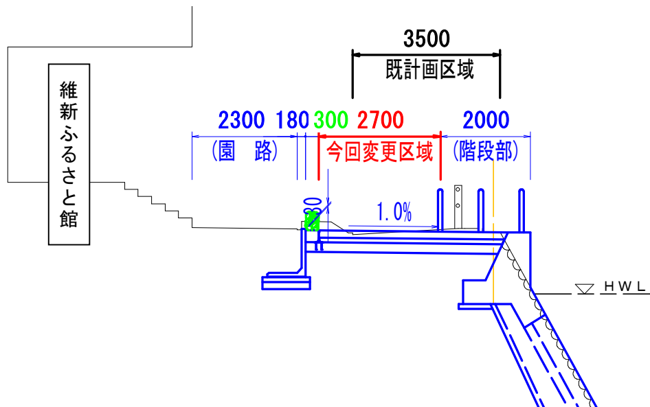
計画横断図(標準部)
