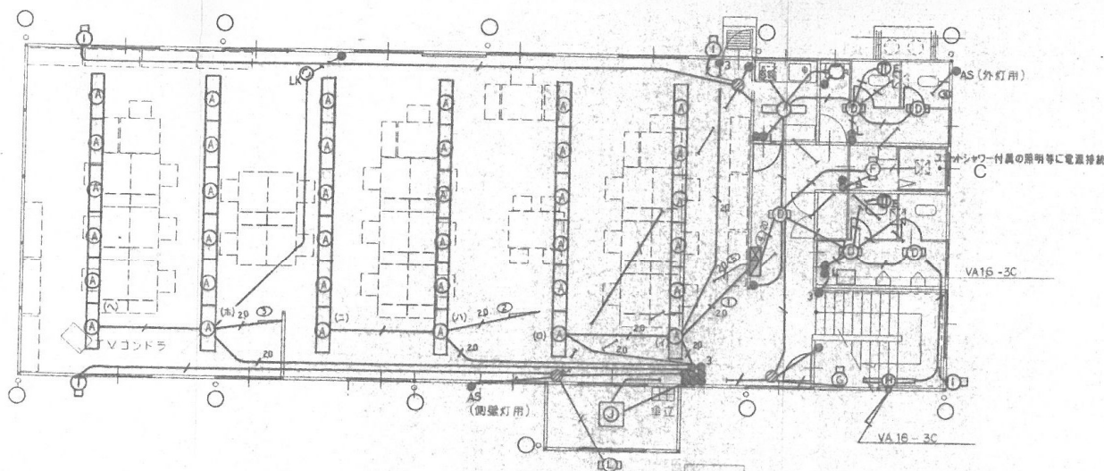
1階電灯設備配線図 S=1/100
