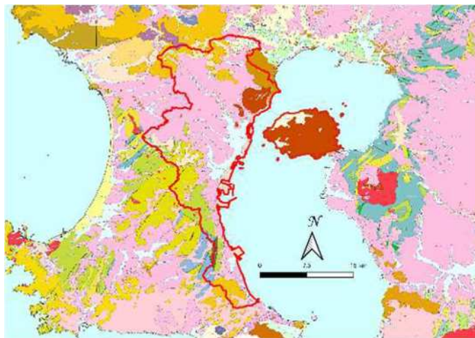
(図 6 : 地質図)
