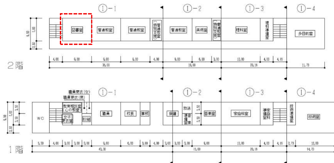
【1-1号棟館内図】
