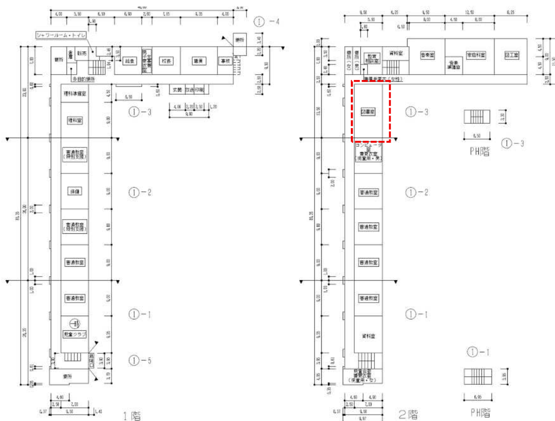
【1-3号棟館内図】
