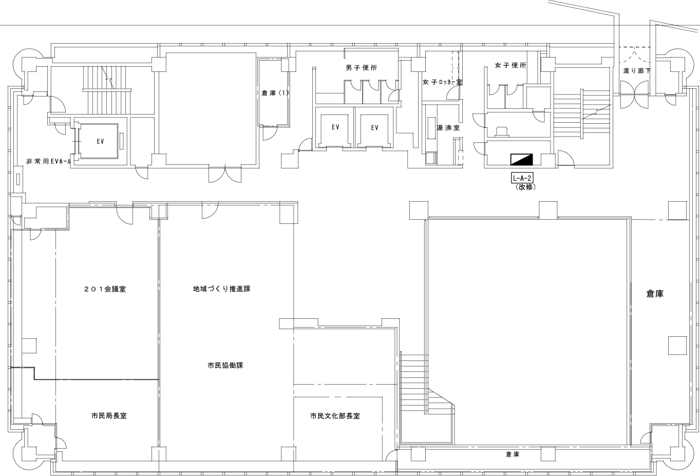
2 階 平 面 図
