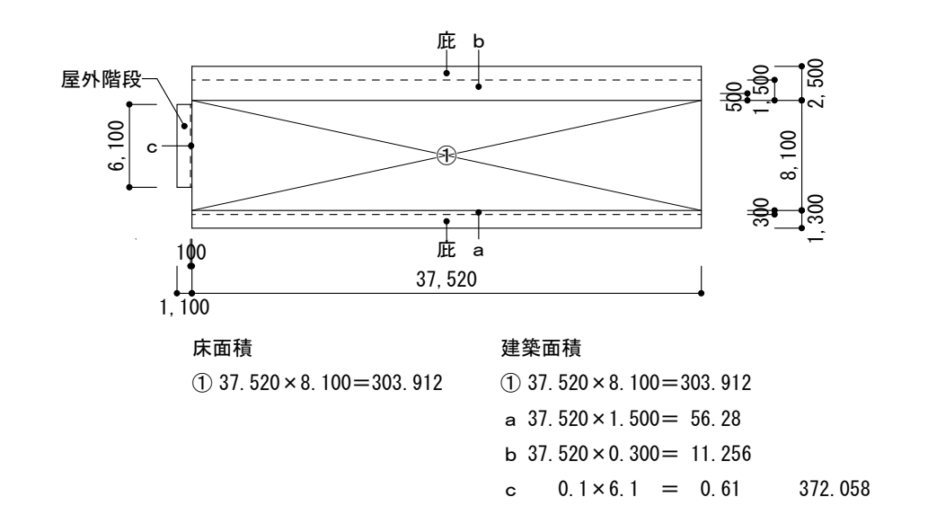
別館1階求積図 1:500
