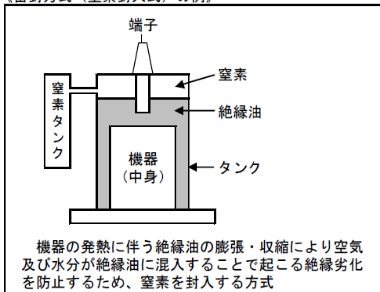
《密封方式（窒素封入式）の例》
