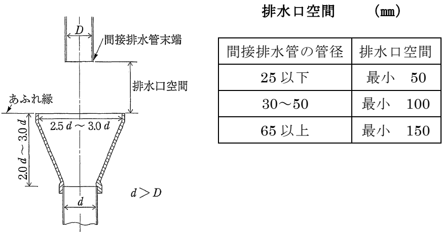
図 3-32 排水口空間
