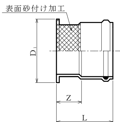
図 3-74 陶管ソケット部にビニル管を接合例
