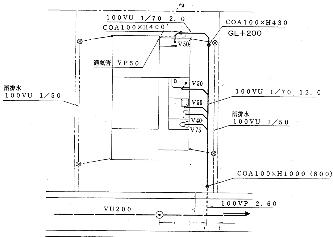
図 3-2 排水設備標準図 (例 1) 平面図縮尺 1/200
