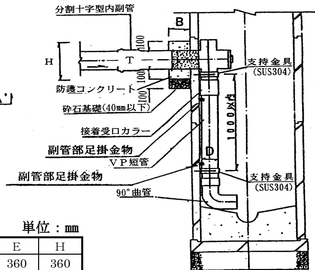
A-A断面图
