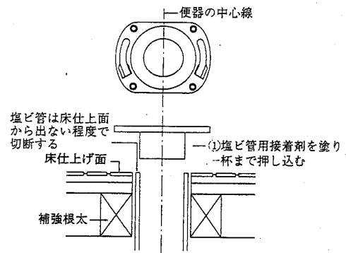
ウ 排水管が硬質塩化ビニル管（樹脂フランジ）の場合の接着例
