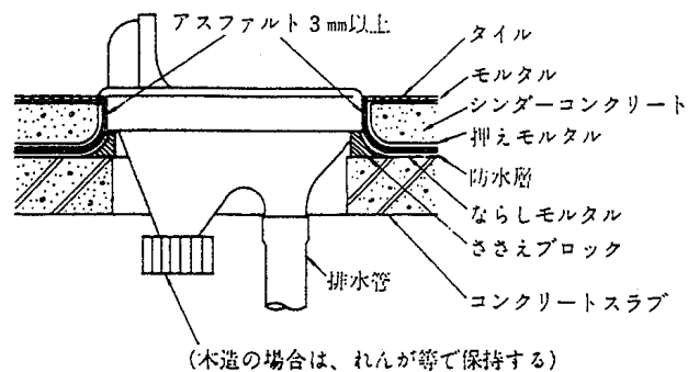
図 3-73 和風大便器の施工例
