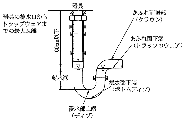
図 3-8 トラップ各部名称例
