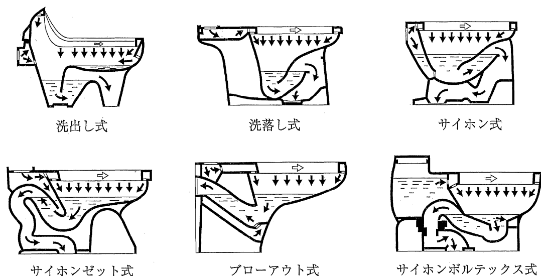
図 3-16 大便器例
