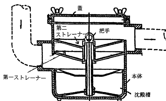
図 3-28-1 プラスト（石膏）阻集器例
