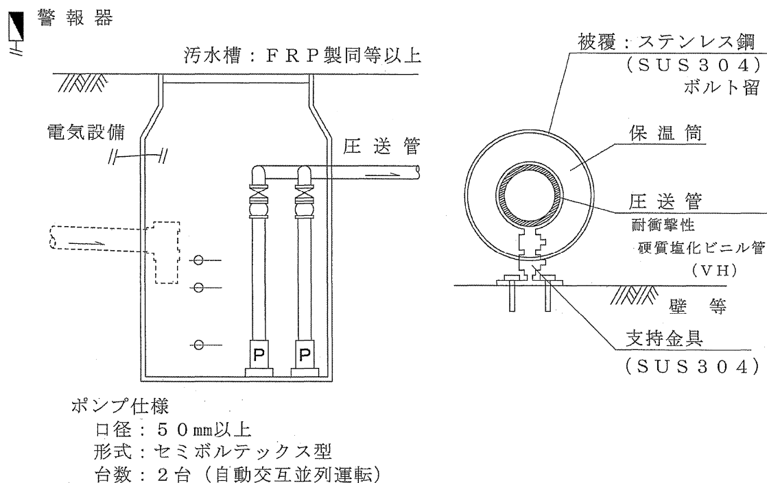
汚水ポンプ施設（ユニット型）例
