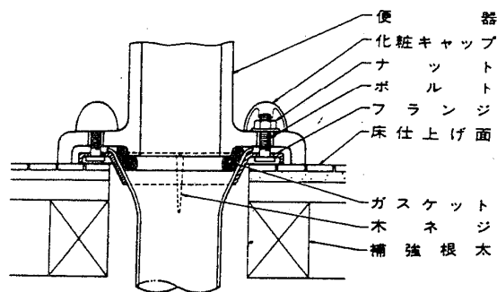
イ 排水管が硬質塩化ビニルの場合
