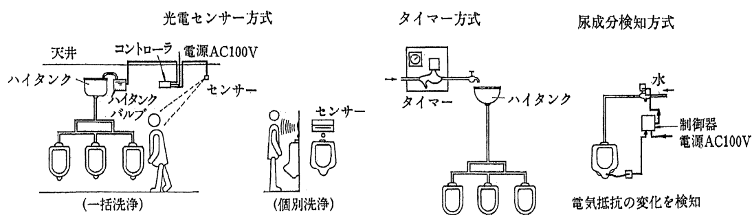
図 3-22 小便器の節水方式例
