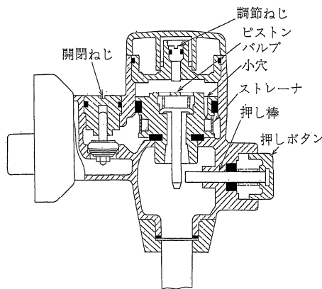
図 3-20 小便器洗浄弁例
