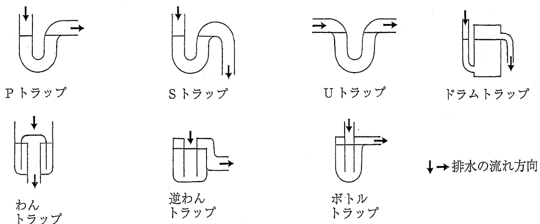
図 3-9 トラップ例
