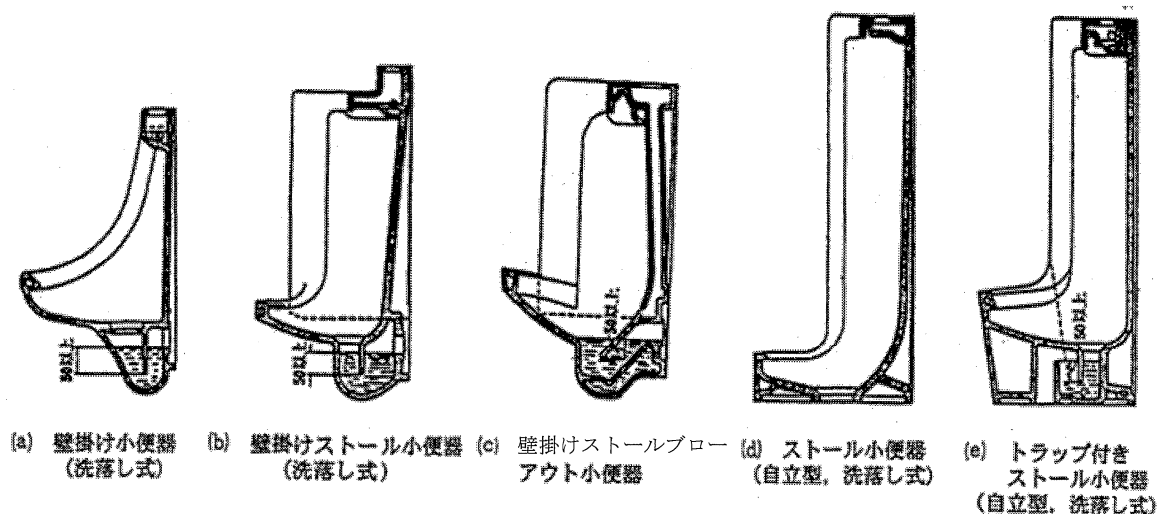
図 3-17 小便器例
