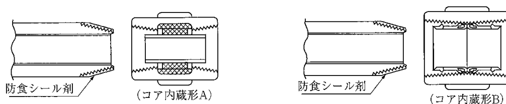
図 3 - 62 ねじ接合例
