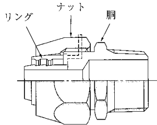
図 3 - 60 メカニカル継手による接合例
