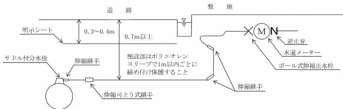
図 3 - 57 ステンレス鋼管の標準配管図例
