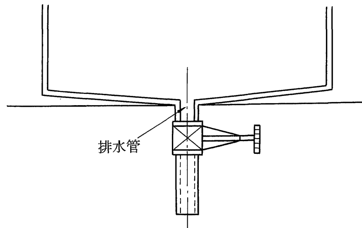
図4-12 高置水槽の排水管例
