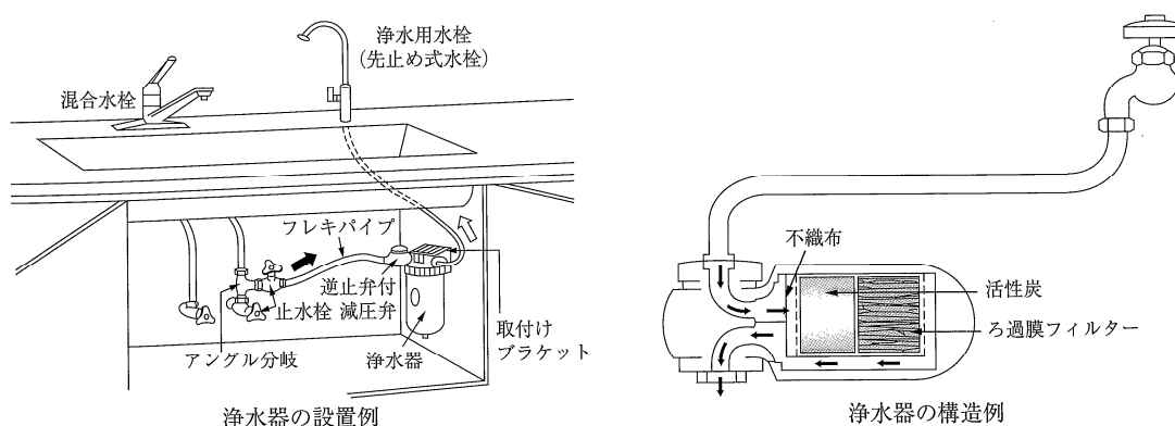
図3-50 浄水器の設置・構造例
