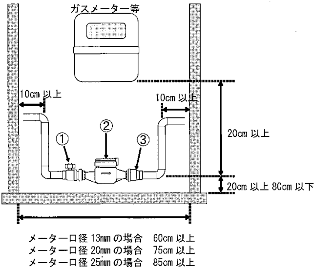
(正面図)
