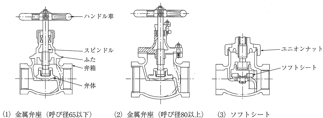
図 3 - 30 玉形弁例
