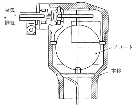
図 3 - 49 吸排気弁例
