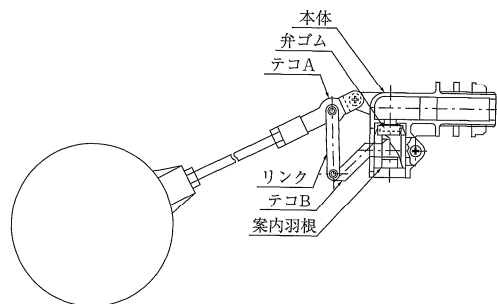
図 3 - 32 - 1 複式ボールタップ(横型) 例
