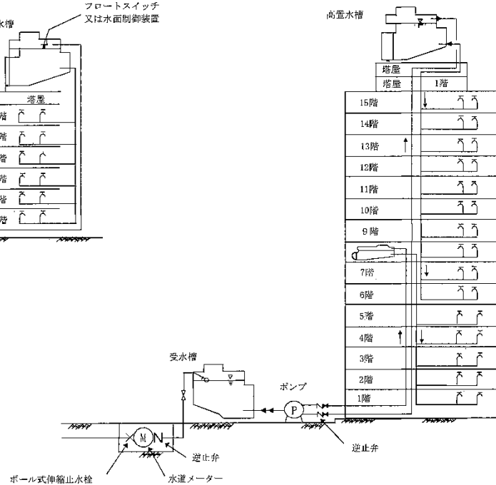
図 3 - 5 多段式高置水槽式例
