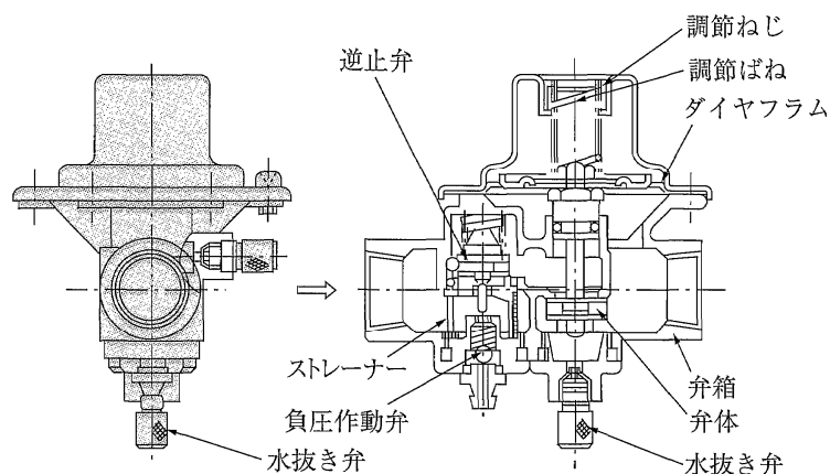
図 3-36 減圧弁例
