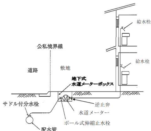
図 3 - 1 直結直圧式例
