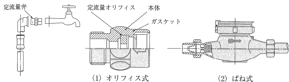
図 3 - 37 定流量弁例
