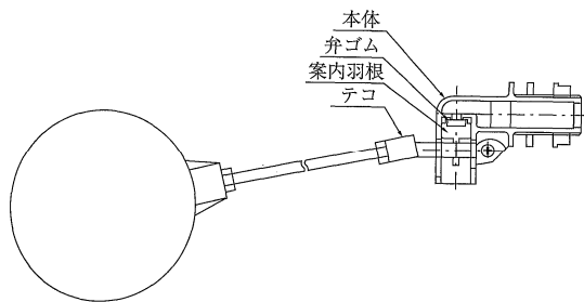
図 3 - 31 単式ボールタップ(横型) 例
