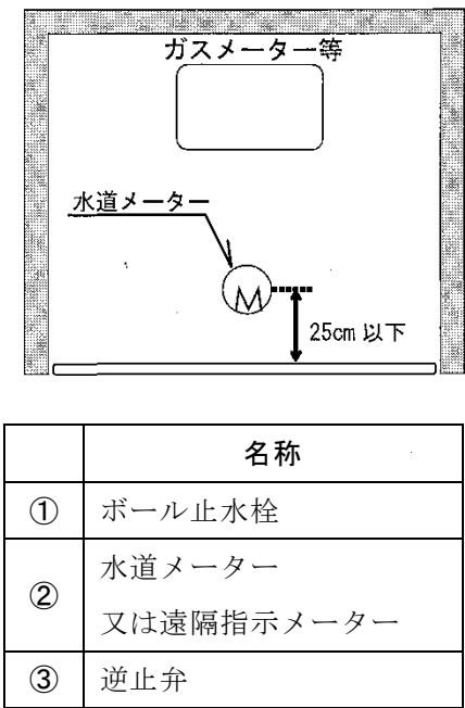
図ー1 メーターユニットを設置する場合 (上面図)
