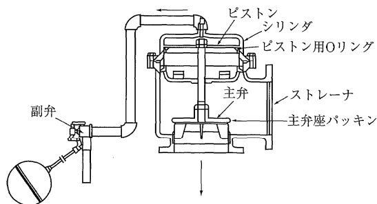
図 3 - 33 副弁付定水位弁例
