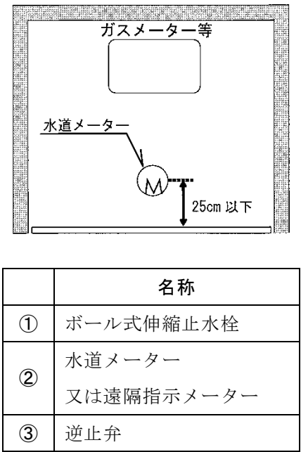
図ー2 メーターユニットを設置しない場合 (上面図)
