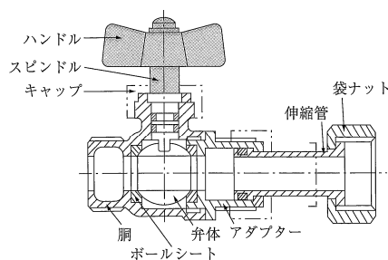
ボール式伸縮止水栓
