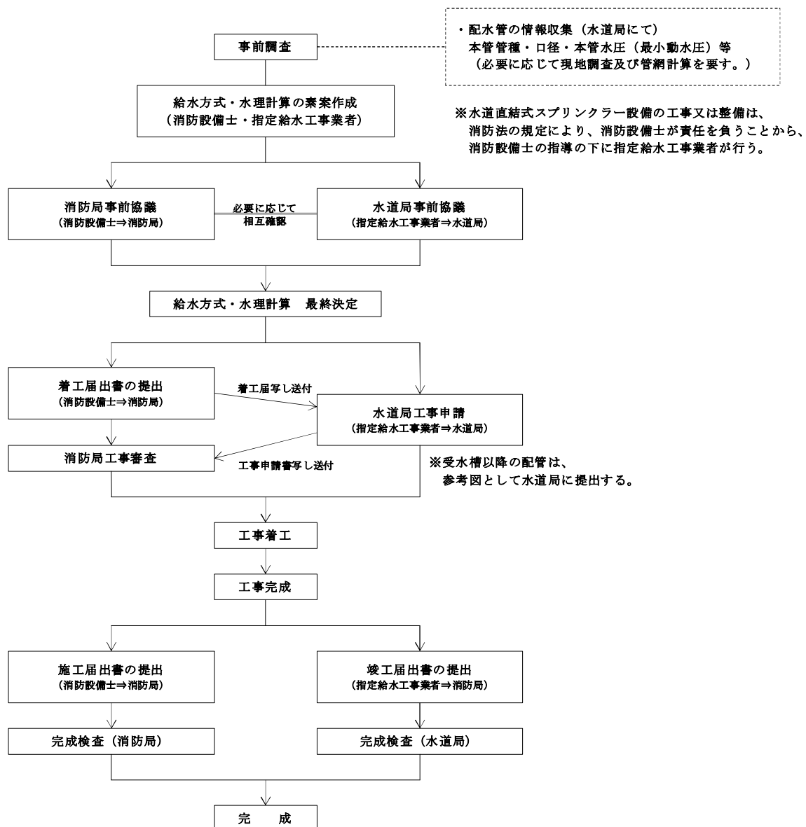
図 1 スプリンクラー設備の設置フロー図
