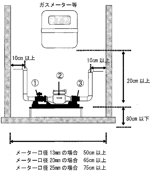
(正面図)
