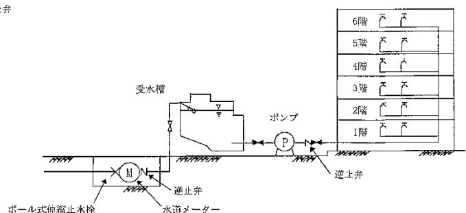
図 3 - 7 ポンプ直送式例
