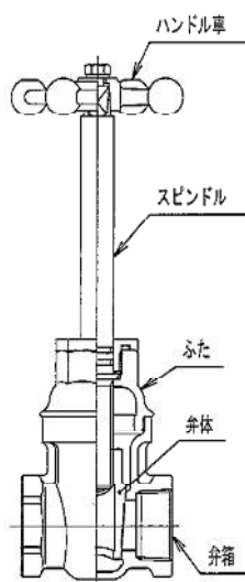
図 3 - 28 仕切弁のつづき(青銅製仕切弁) 例
