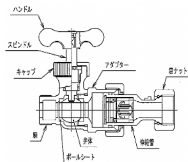
逆止弁付伸縮ボール止水栓
