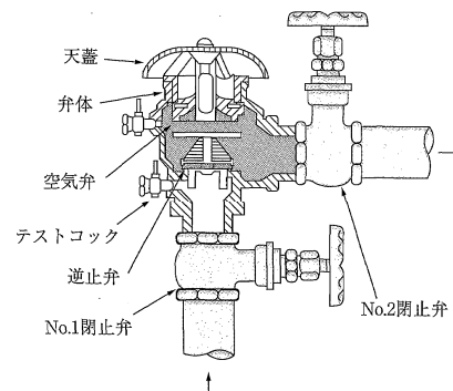
図 3 - 46 圧力式例
